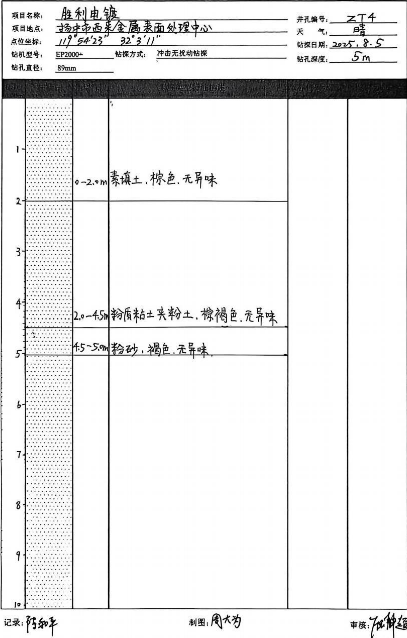
钻孔柱状图
