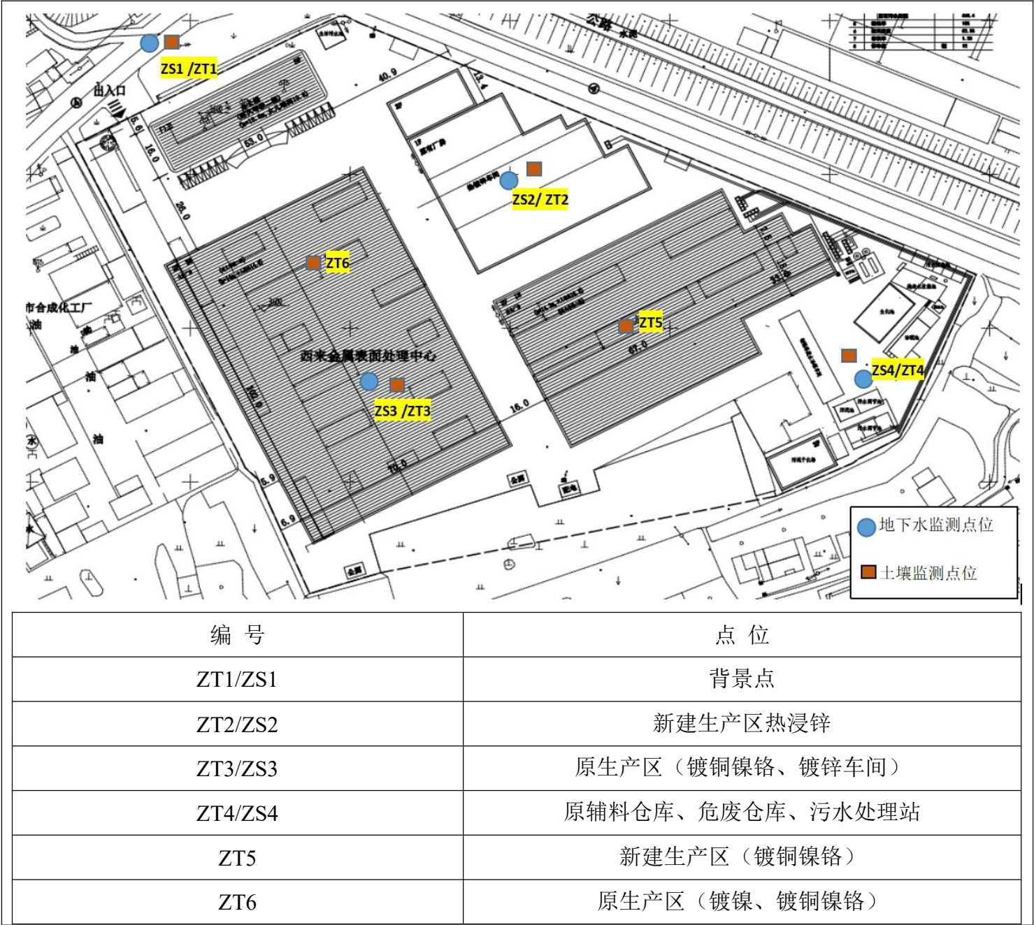
图 6-1 监测点位平面布置图
