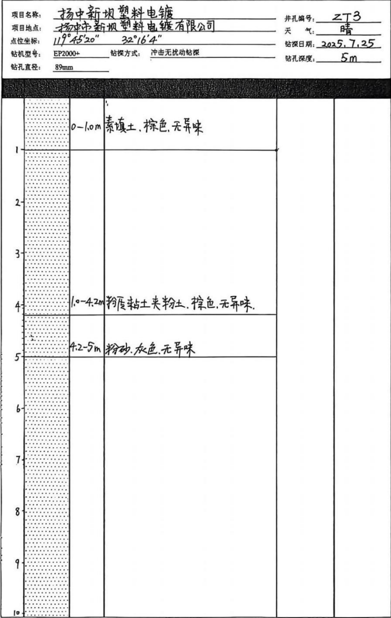
钻孔柱状图
