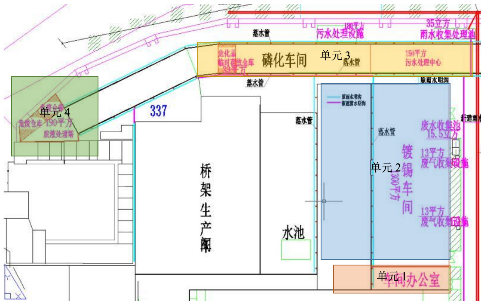
图 4.3-1 企业平面布置中重点设施分布情况
