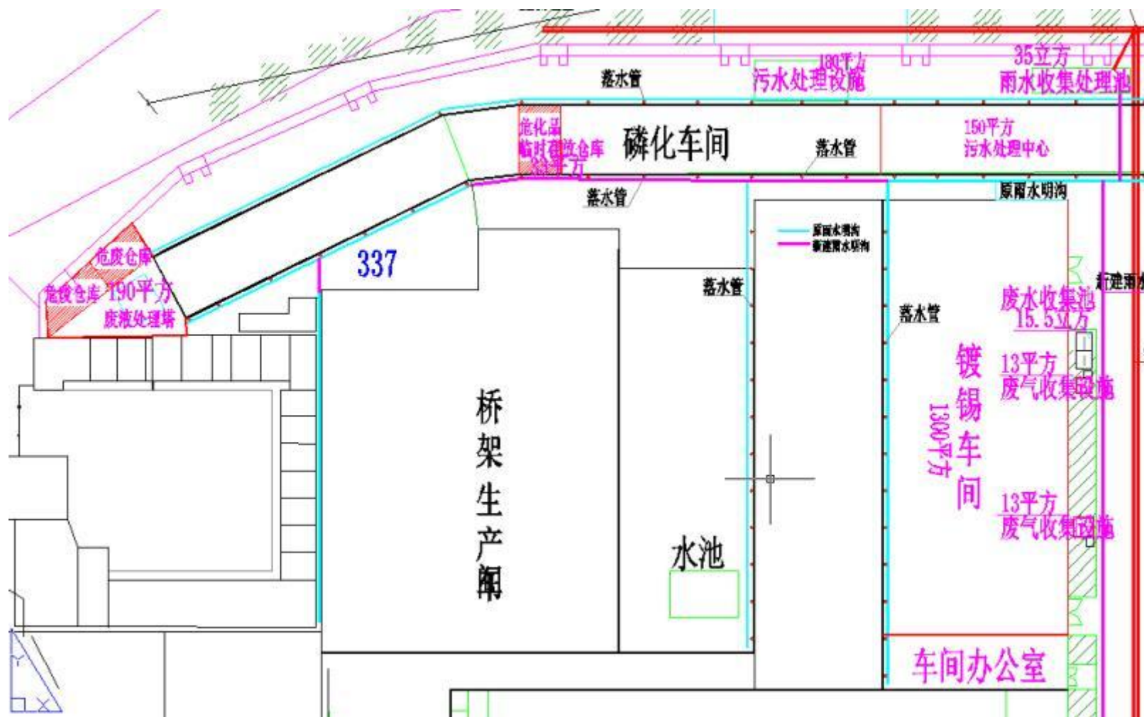
图 4.2-1 企业总平面布置图
