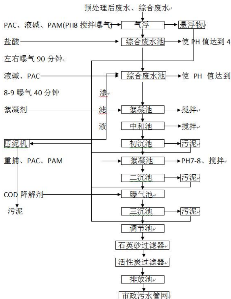
图 4.1-1 综合废水处理流程
