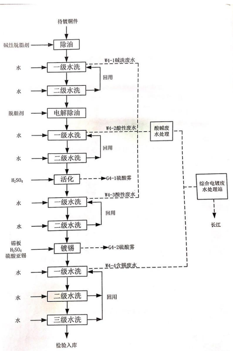
图 4.1-3 铜件镀锡自动线工艺流程
