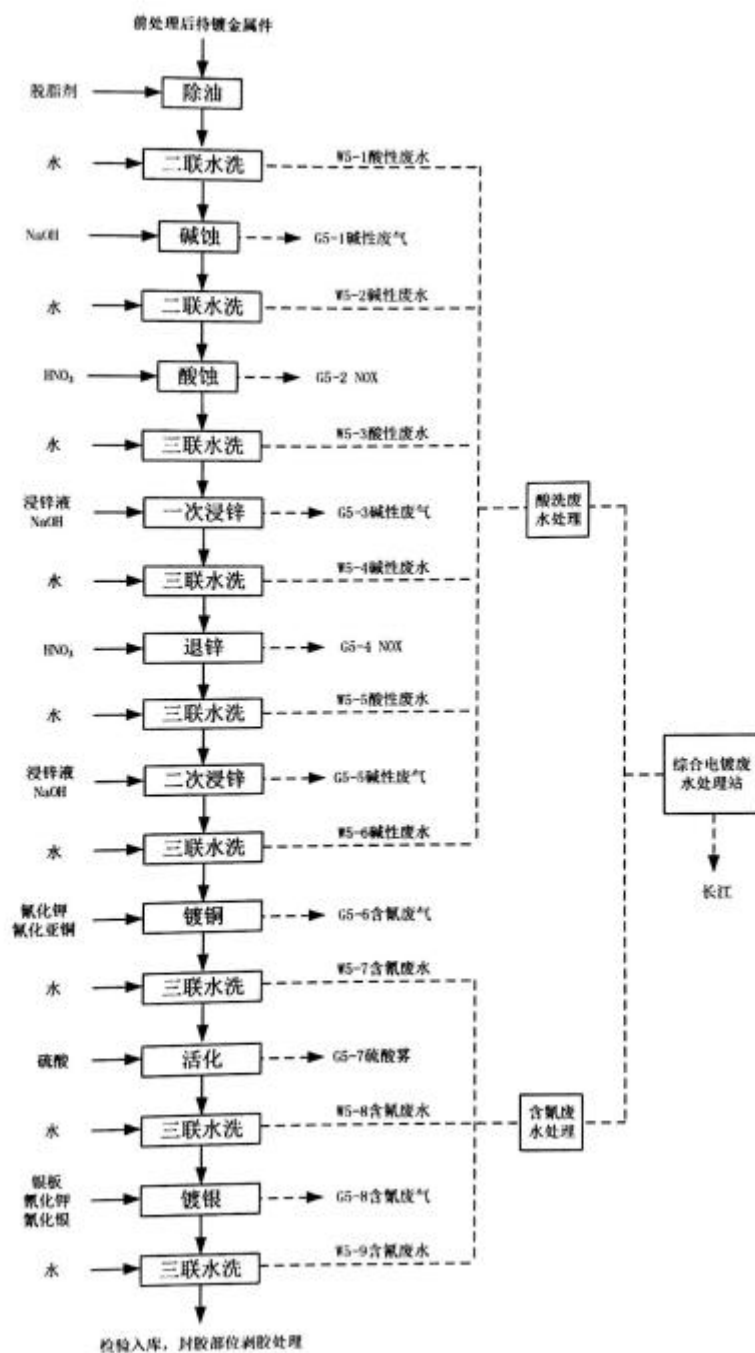
图 4.1-4 GIS 镀银工艺流程
