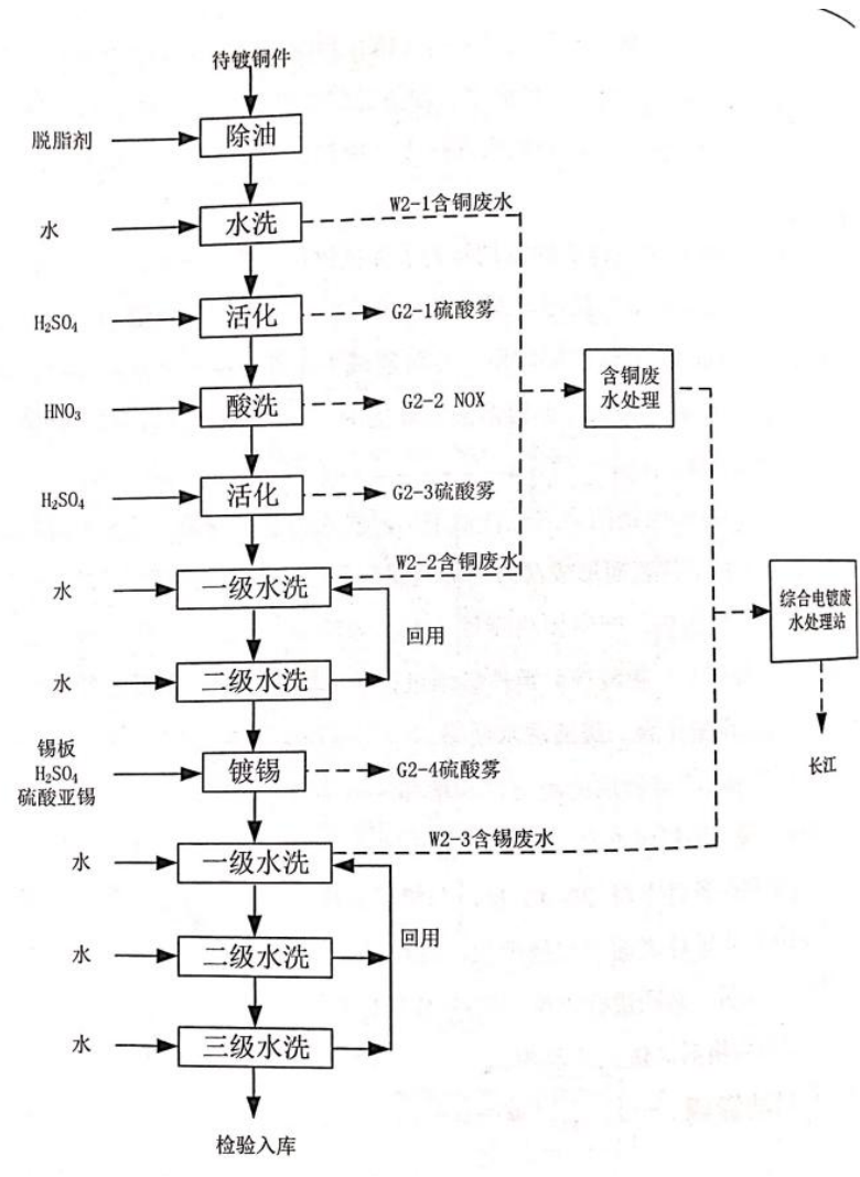
图 4.1-2 铜件镀锡半自动线工艺流程
