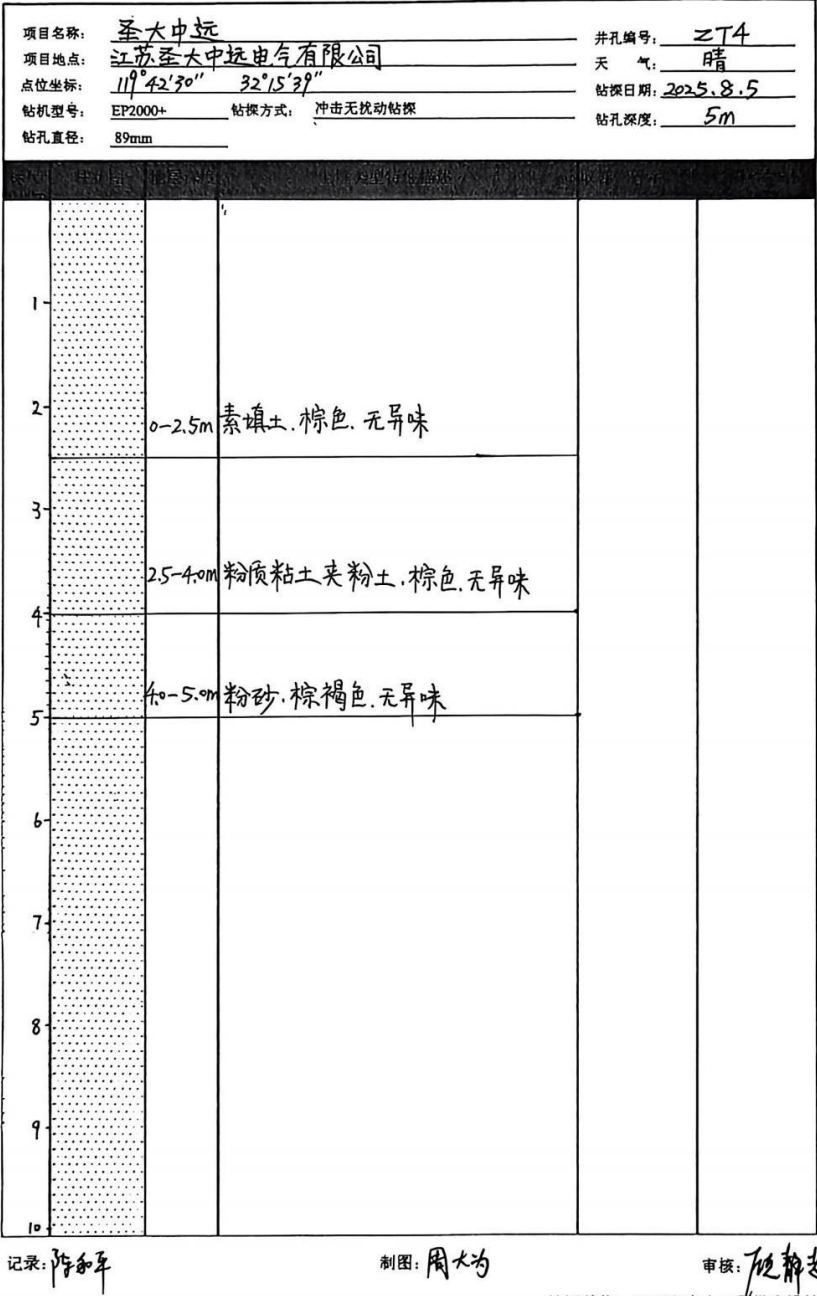
钻孔柱状图
