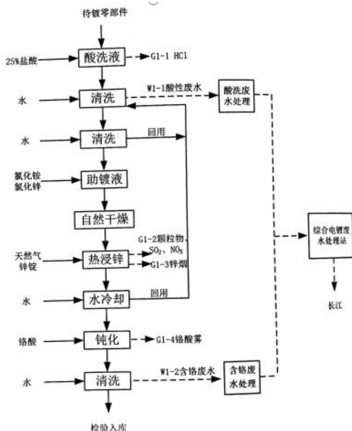
图 4.1-1 热浸锌工艺流程
