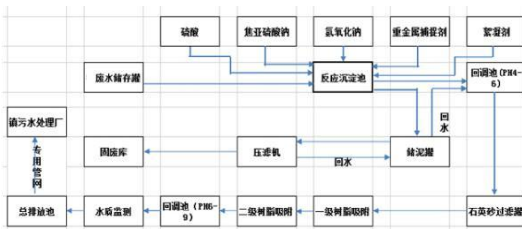
含铬废水处理系统
