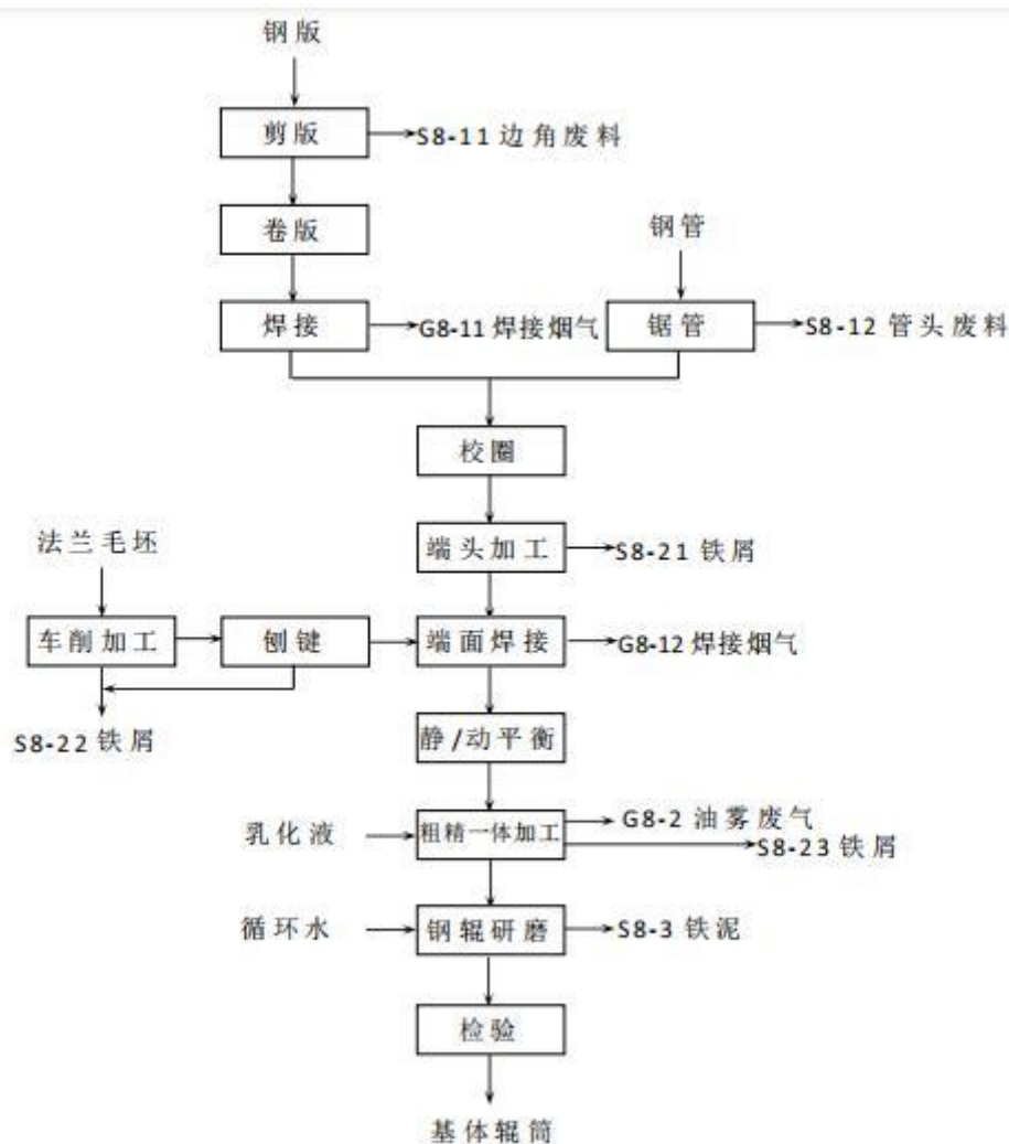
机辊筒机加工生产工艺流程及产污环节图
