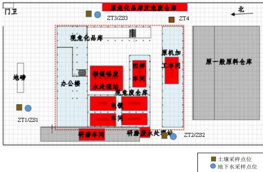
图 6-1 监测点位平面布置图
