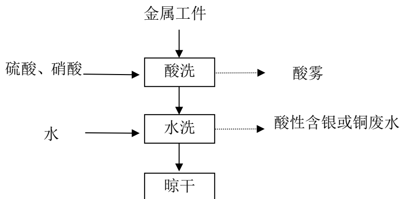
图4.1-4 退镀线工艺流程及产污环节图
