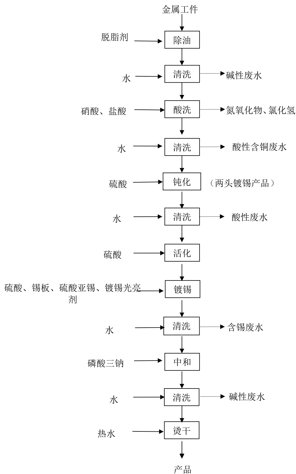
图4.1-1 镀锡自动生产线工艺流程及产污环节图
