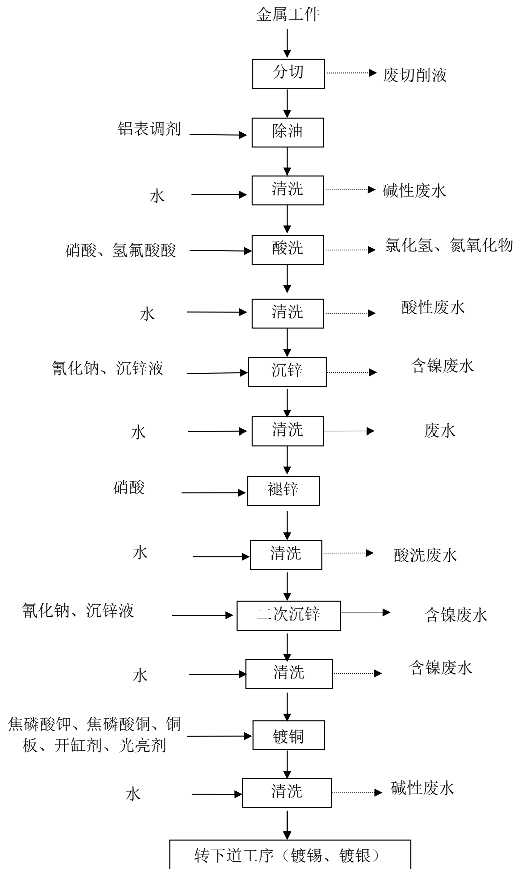
图4.1-3 铝排镀铜生产线工艺流程及产污环节图
