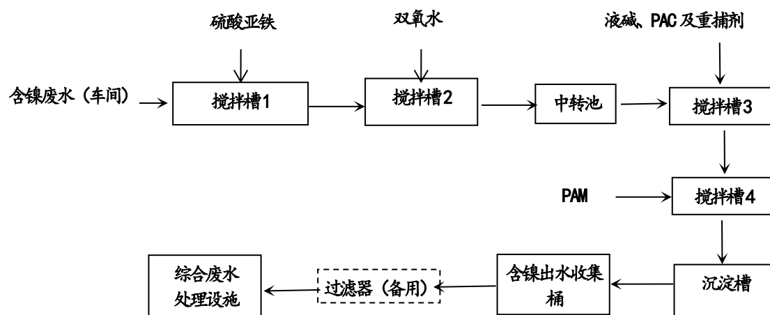
图4.2-2 含镍废水处理流程图
