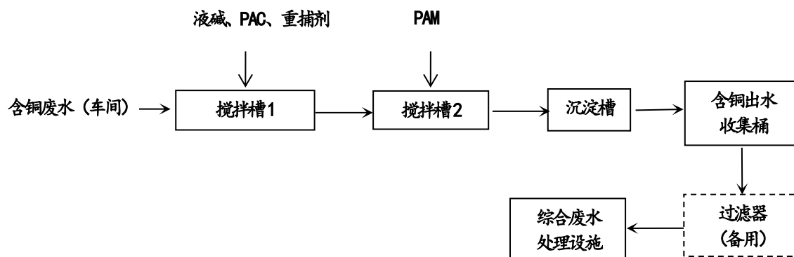
图4.2-3 含铜废水预处理流程图
