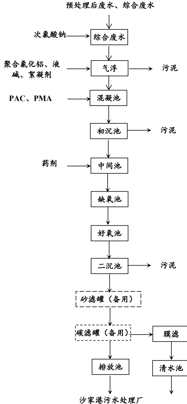
图4.2-4 综合废水处理流程图
