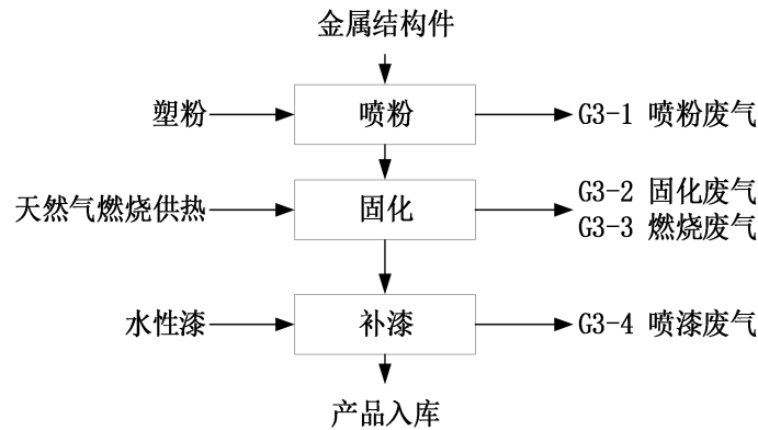
图4.1-7 喷涂生产线工艺流程及产污环节图
