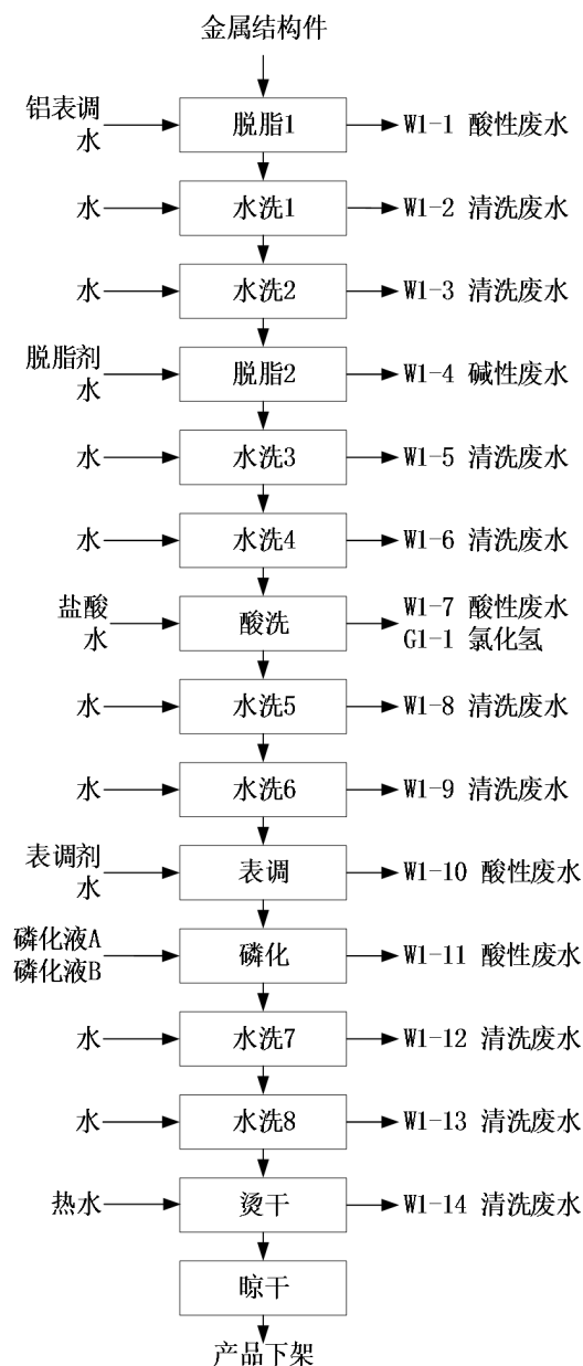
图4.1-5 酸洗生产线工艺流程及产污环节图
