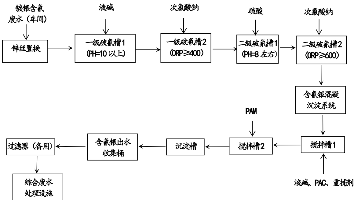
图4.2-1 含氰废水处理系统处理流程图
