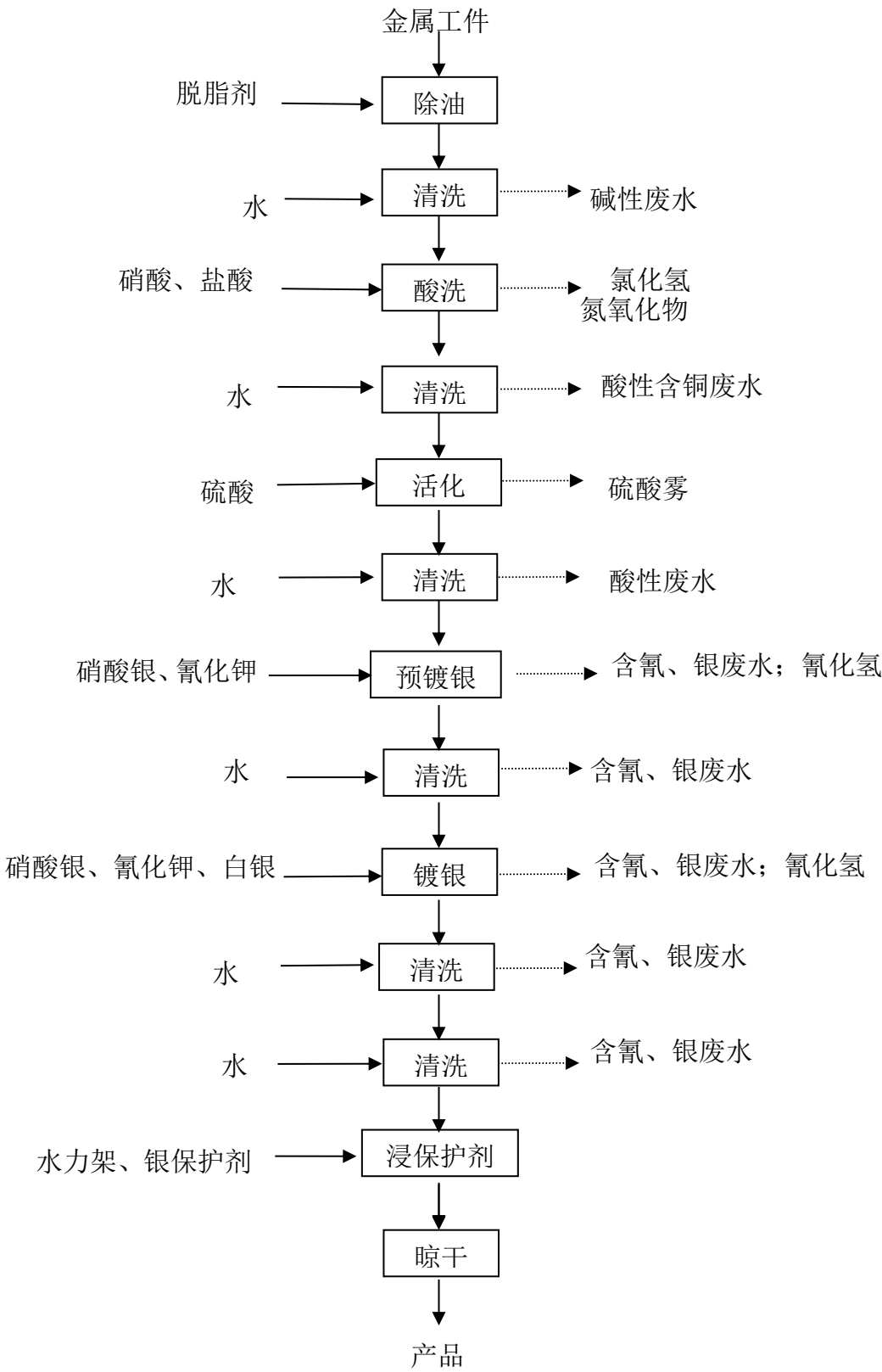
图4.1-2 镀银生产线工艺流程及产污环节图
