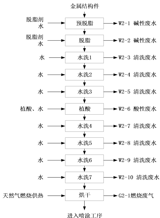
图4.1-6 喷淋生产线工艺流程及产污环节图
